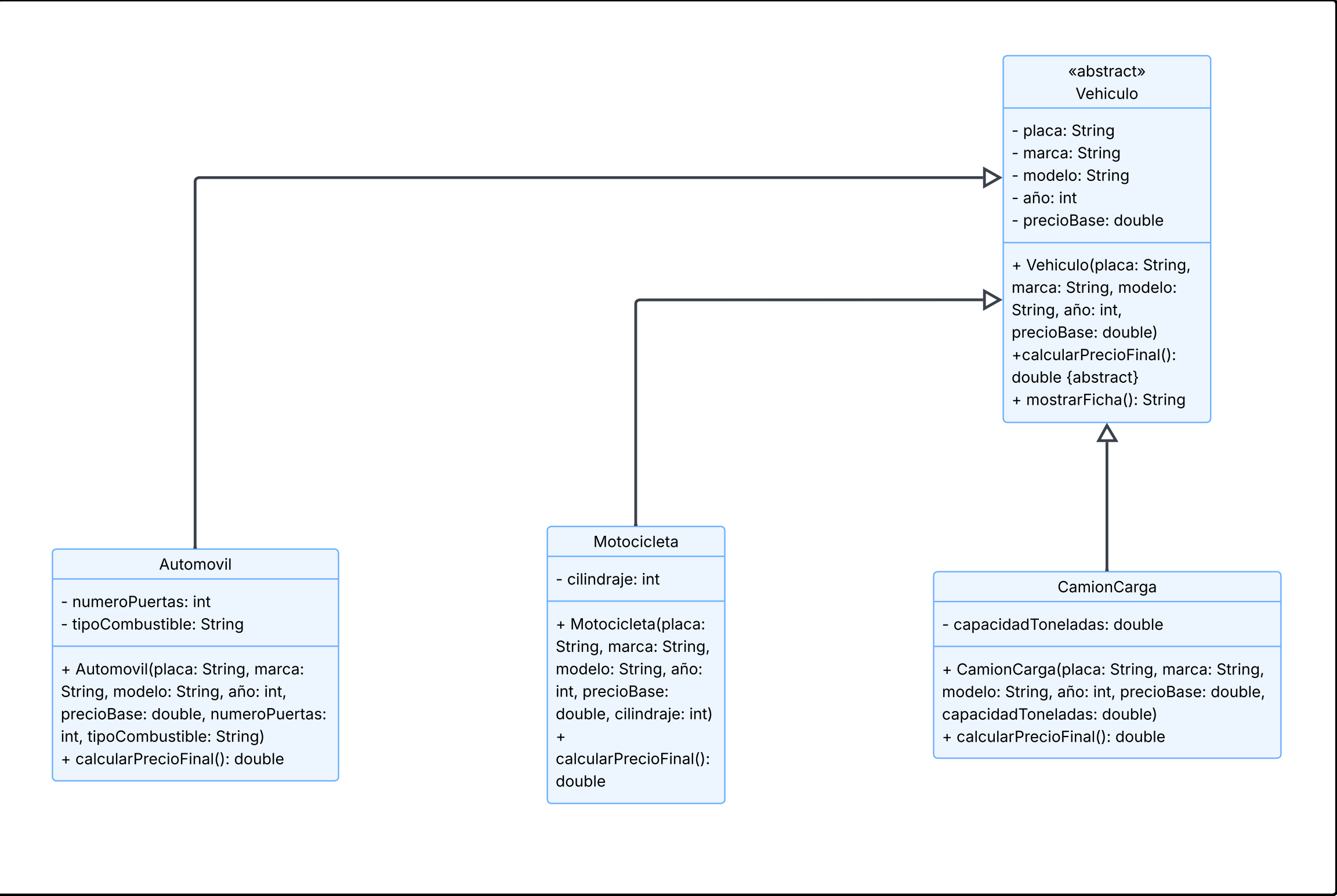
Diagrama de Clases UML: Vehiculo y Subclases
